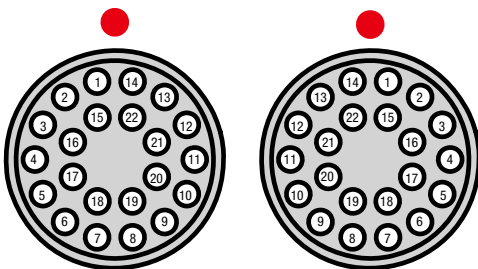
SE2L-H05LPC Pin No.
